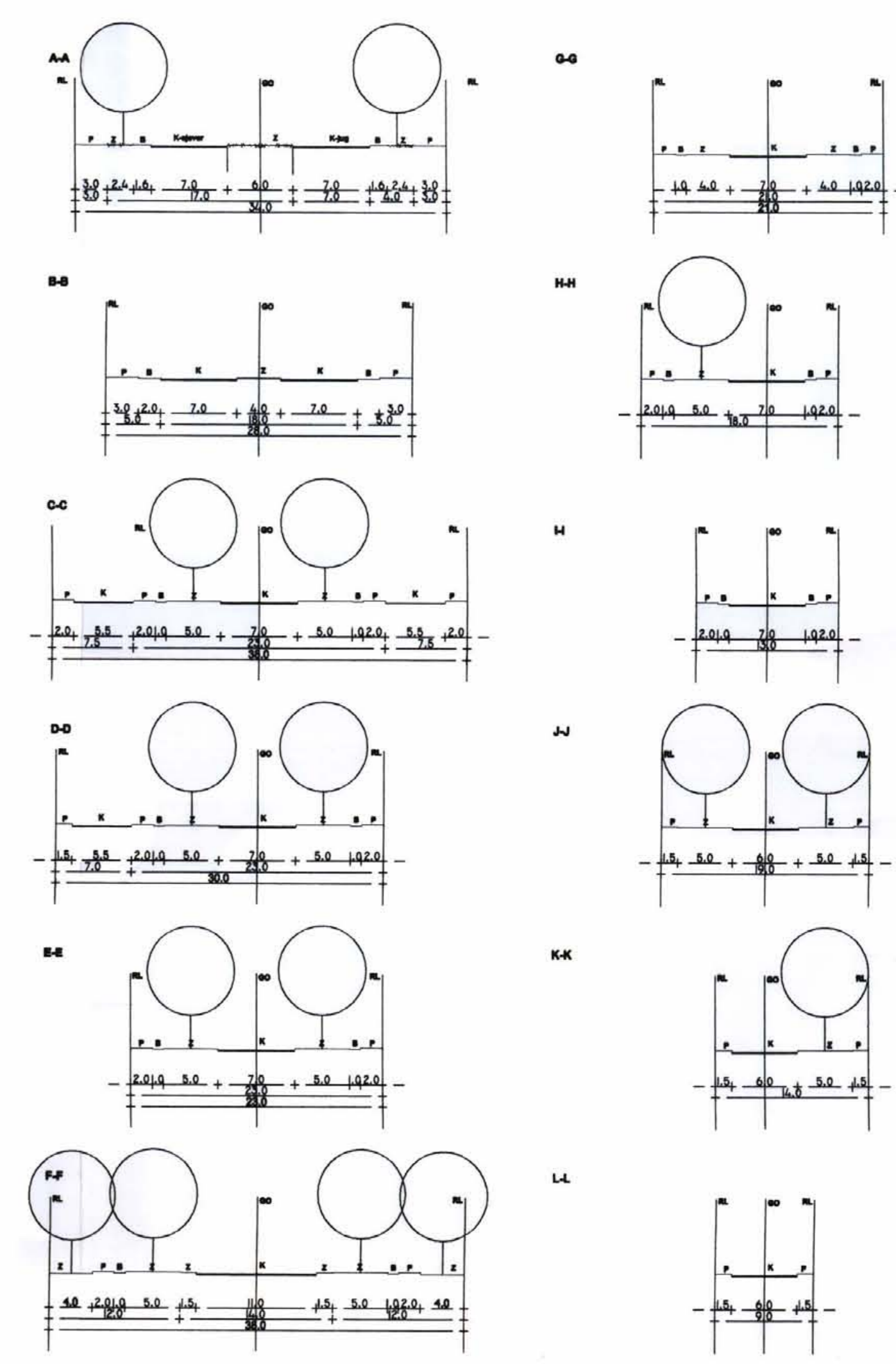
PROFILI CESTOVNIH KORIDORA MJ. 1:400
